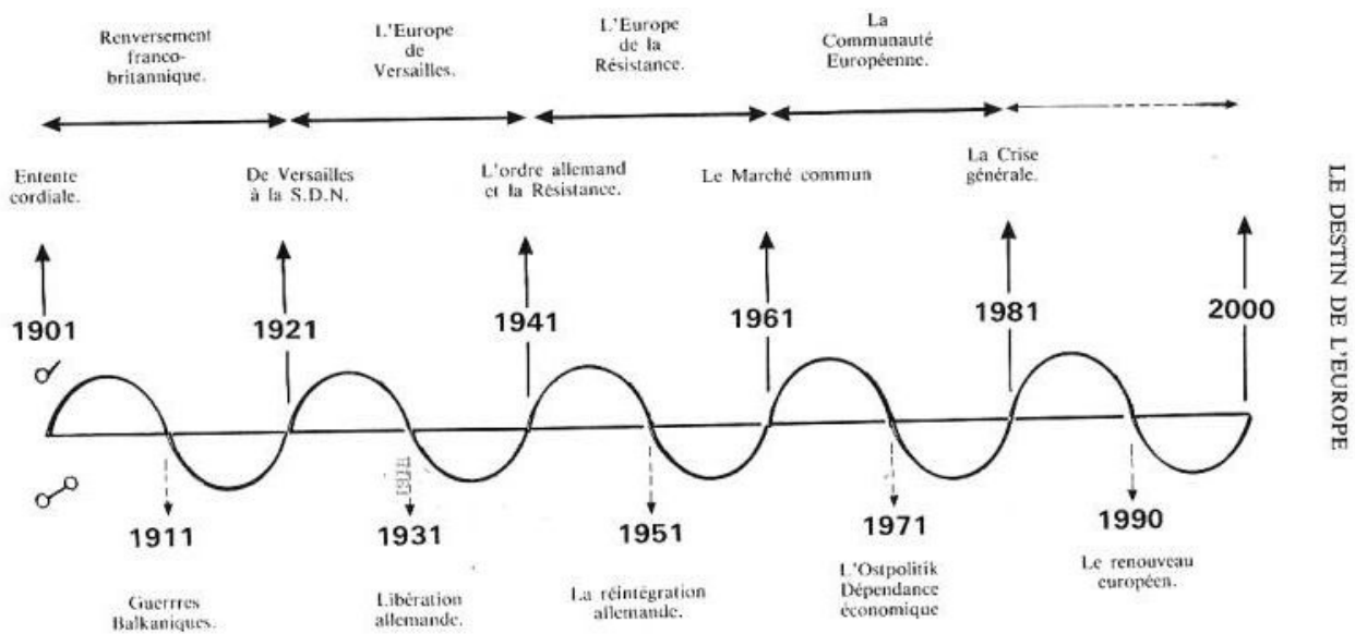
Le sorti dell'Europa e l'andamento del ciclo Giove-Saturno
