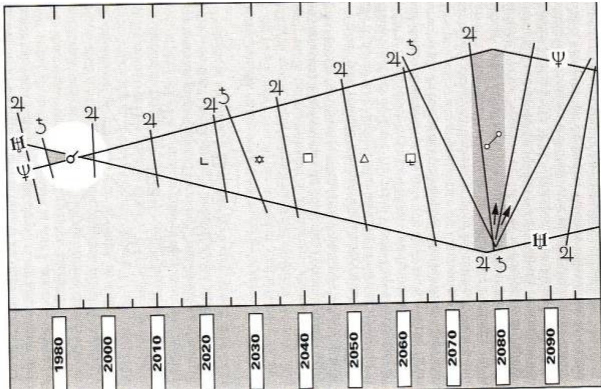
Ciclo Urano-Nettuno, e sue interferenze da parte di Giove e Saturno
