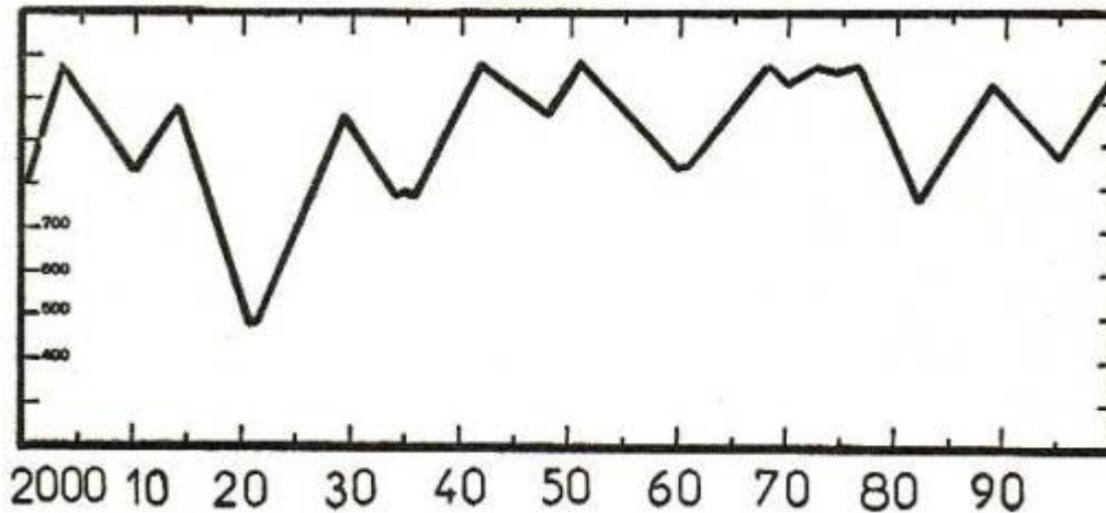
Indice Ciclico Planetario per il XXI secolo
